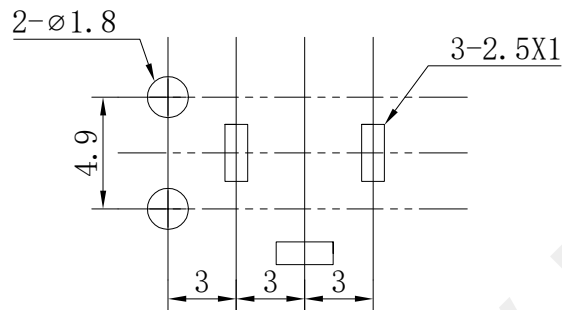
线路板开孔尺寸 P.C.B LAYOUT
